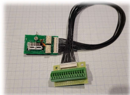
Med termineringskort för smidig inkoppling av alla funktioner
