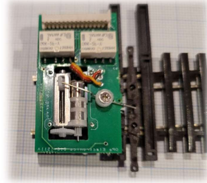
Servot monterat under en PECO-växel
