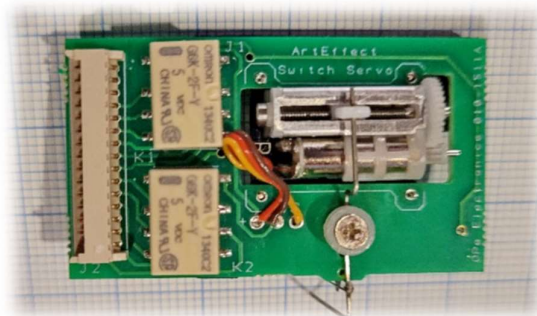
Servo med relä-återkoppling av växels lägen
