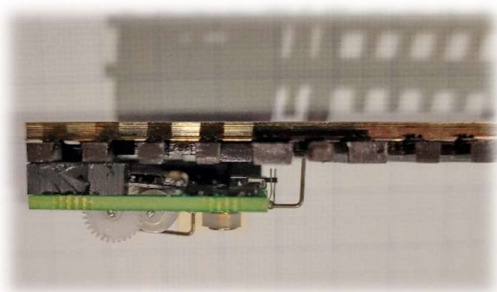
Servot monterat under växeln och sett från sidan
